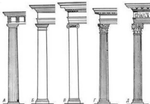
А – дорический ордер; Б – тосканский ордер; В – ионический ордер; Г – коринфский ордер; Д – композитный ордер.
