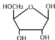
В) Рибоза
