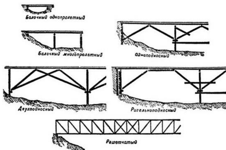
Основные системы деревянных мостов
