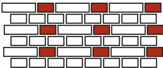
А) Голландская кладка;
