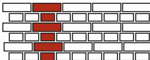
Г) Крестовая кладка.
