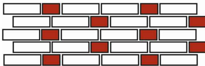
Б) Цепная кладка;
