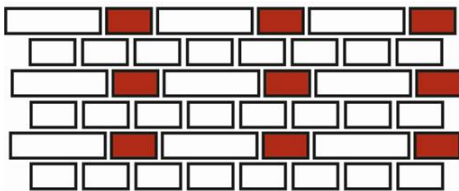
А) Голландская кладка;
