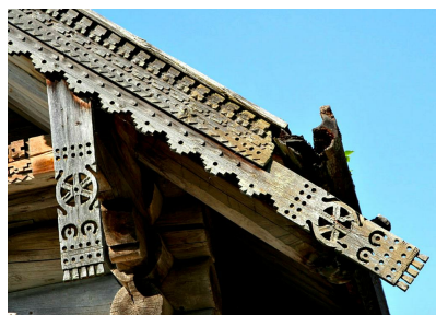
Г) Причелина с резьбой.
