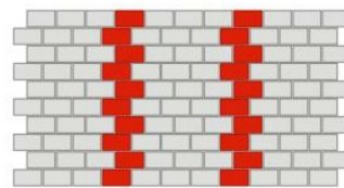
ЛОЖКОВЫХ РЯДОВ
