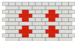
КРЕСТОВАЯ ПЕРЕВЯЗКА ТИП 1
