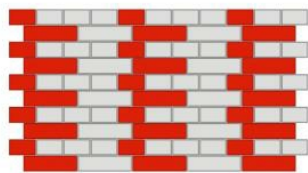
БЛОЧНАЯ ПЕРЕВЯЗКА
