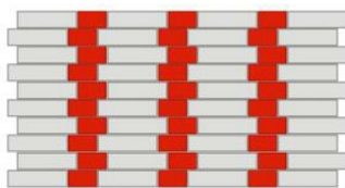
ГОТИЧЕСКАЯ ПЕРЕВЯЗКА
