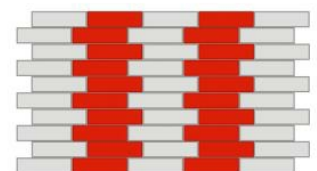
ЛОЖКОВАЯ ПЕРЕВЯЗКА - СМЕЩЕНИЕ НА 1/3 КИРПИЧА
