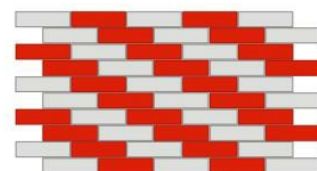
ЛОЖКОВАЯ ПЕРЕВЯЗКА - СМЕЩЕНИЕ НА 1/4 КИРПИЧА
