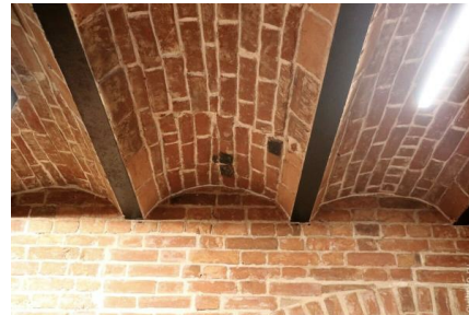
Б) Своды Монье;
